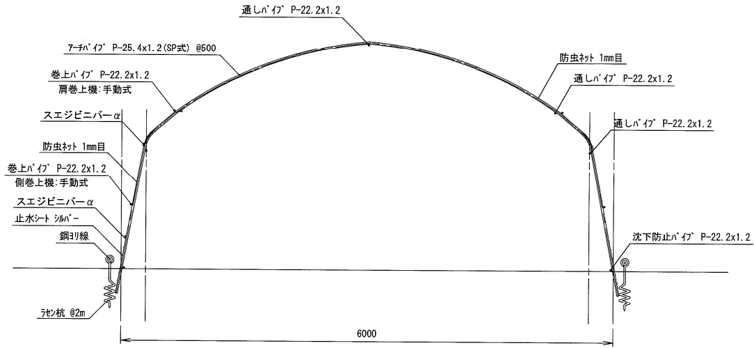
矩計図
