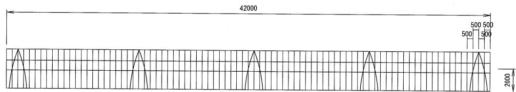
側立面図 S=1/200
