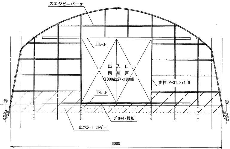
妻面図
