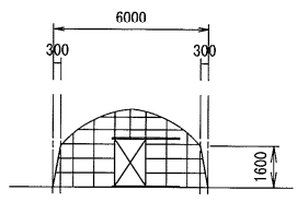
1 通り 妻立面図 S=1/200
