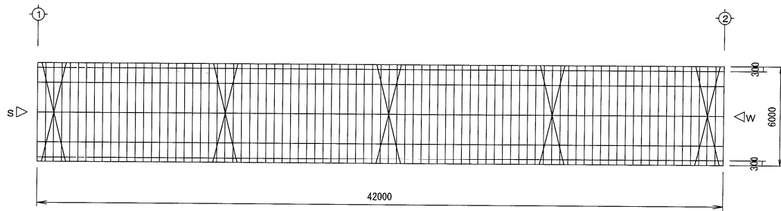
平面図 S=1/200
