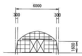
2 通り 妻立面図 S=1/200
