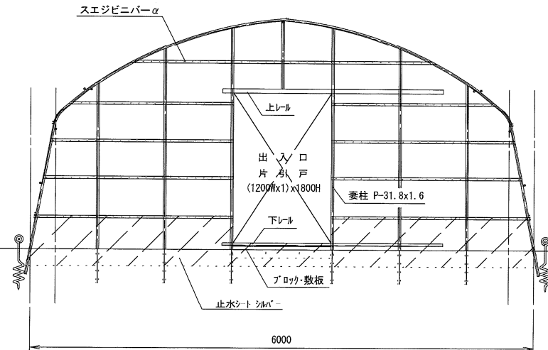
妻面図
