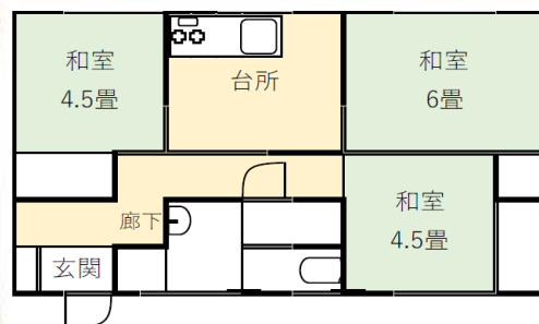
間取り (3K)
